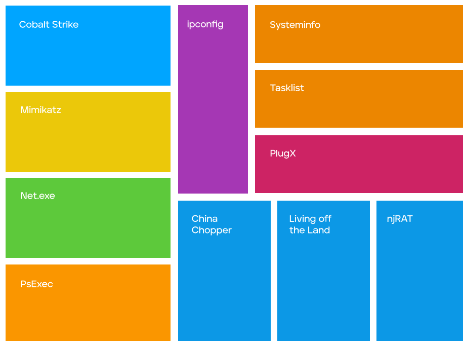
Figure 3. Cobalt Strike (34 %) a été l'outil malveillant le plus souvent détecté au 3 e trimestre 2021, suivi de Mimikatz (27 %), Net.exe (26 %) et PsExec (20 %). La suite d'attaques Cobalt Strike exploitée par des pirates à la solde d'États a été identifiée dans plus d'un tiers des activités APT.
